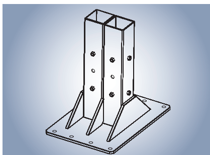
Aufschraubständer Reihenanlage (verzinkt und pulverbeschichtet)
