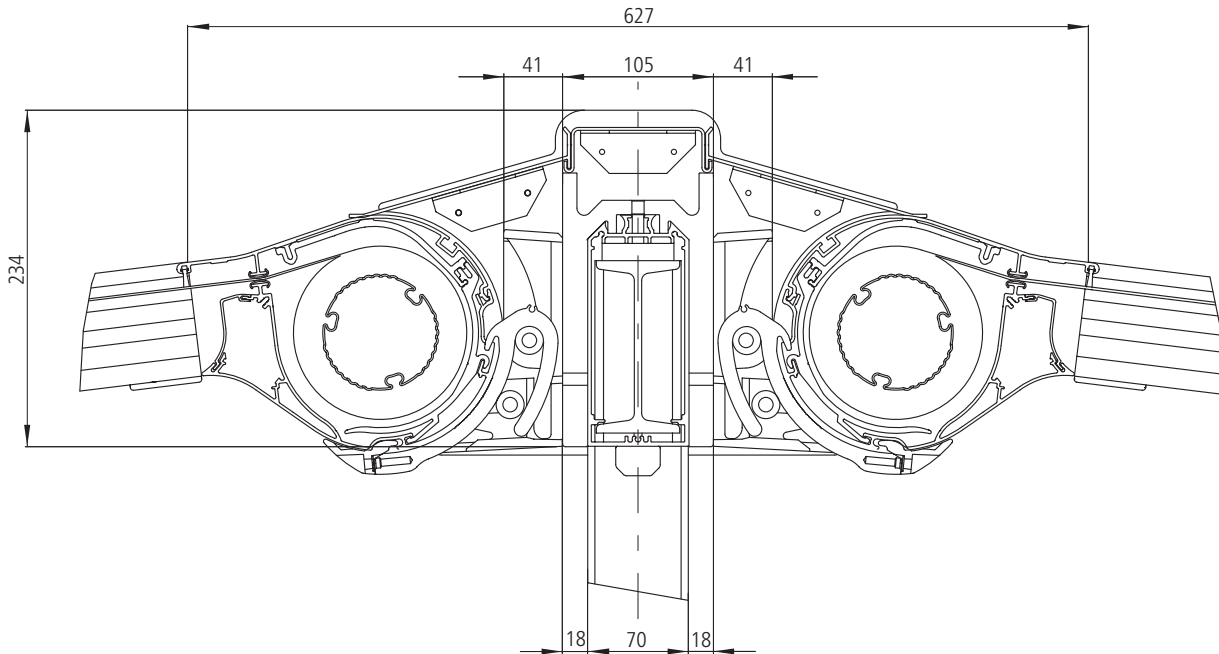
Schnittzeichnung Duofix mit Plaza Viva
