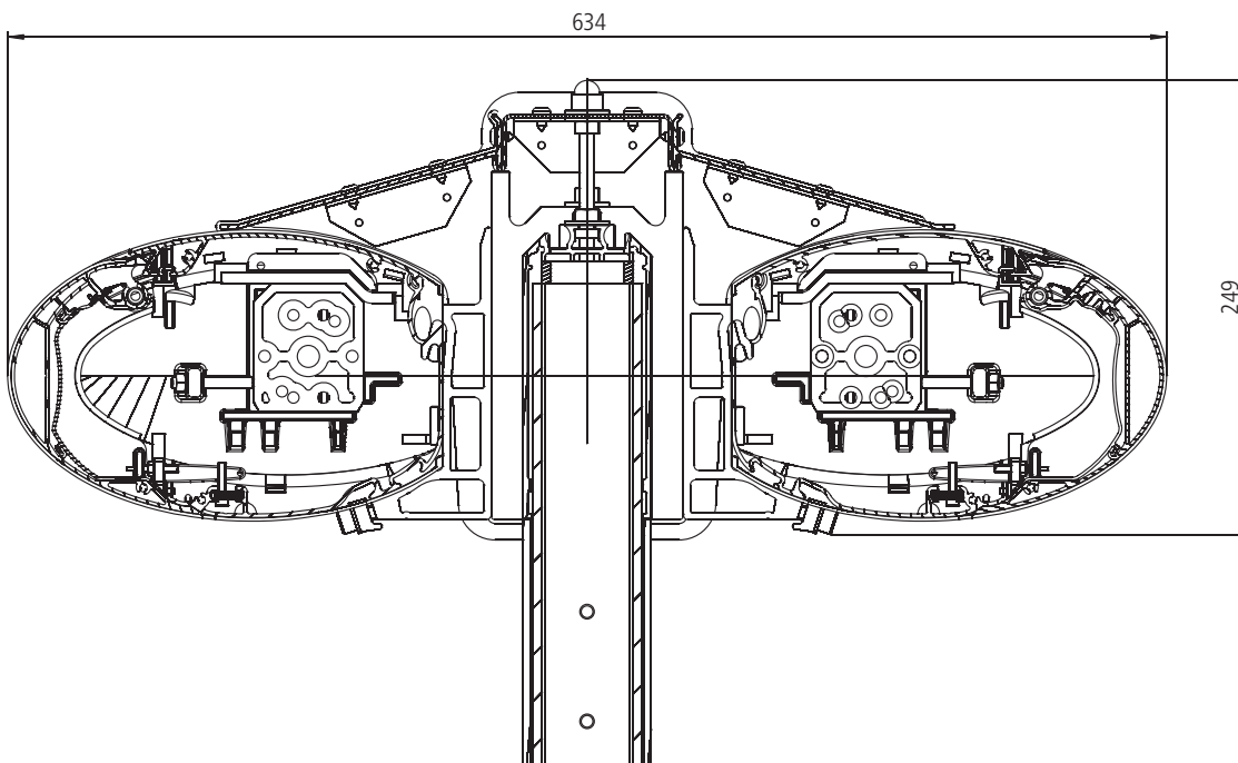
Schnittzeichnung Duofix mit Opal Design II
