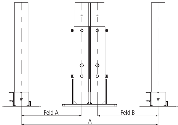
Beispiel einer Aufstelloption: Aufschraubständer bei Mehrfeldanlagen
