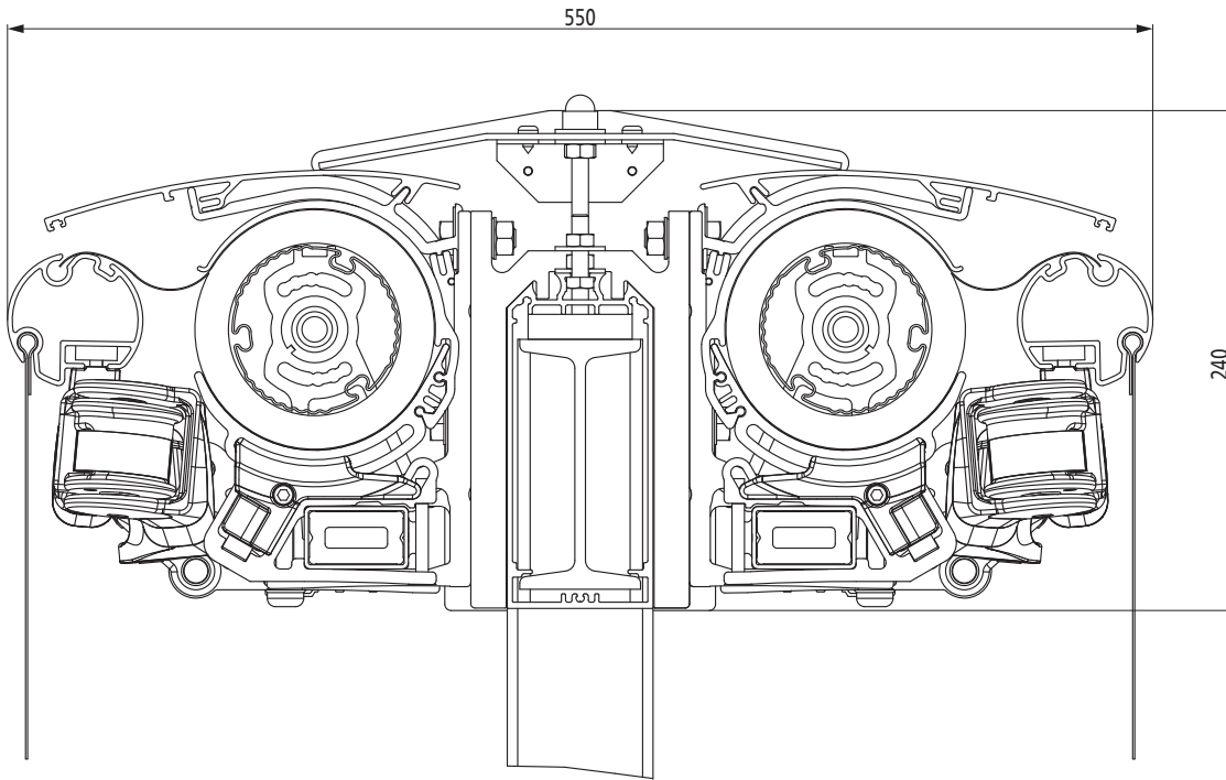
Schnittzeichnung Duofix mit Topas II mit Dach
