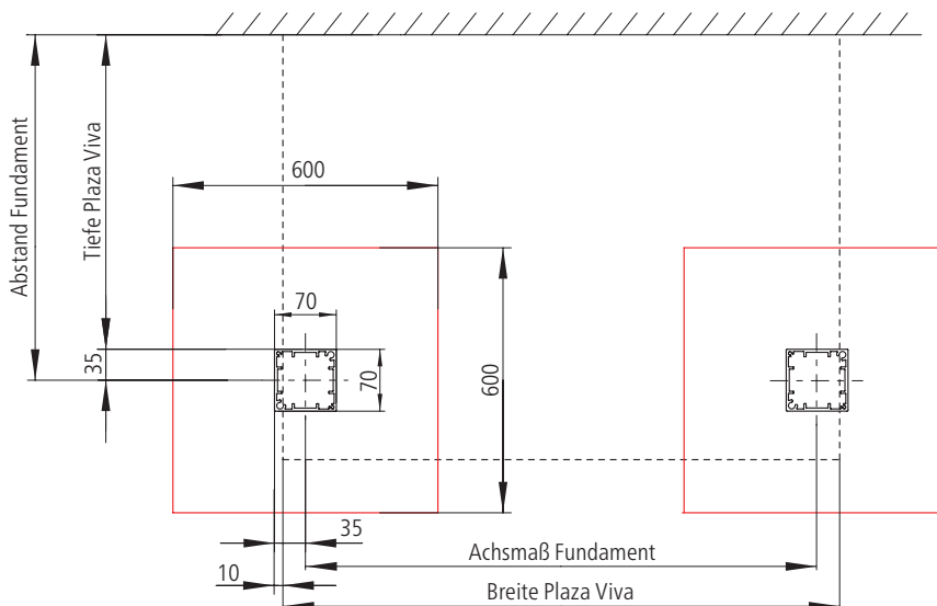
Pfosten Fundament-Plan
